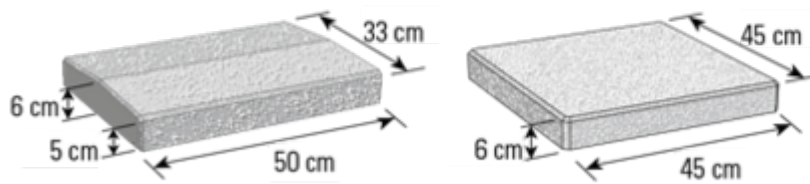
Abdeckplatte
