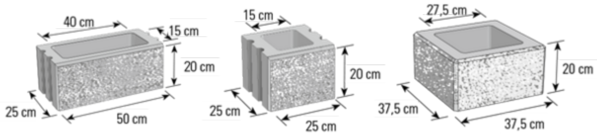
Grundelement
