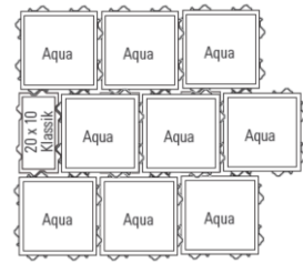
Pose à joints décalés
