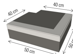
Außenecke 90° (für Stufenbreite 40 cm)
