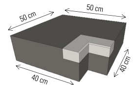
Innenecke 90° (für Stufenbreite 40 cm)
