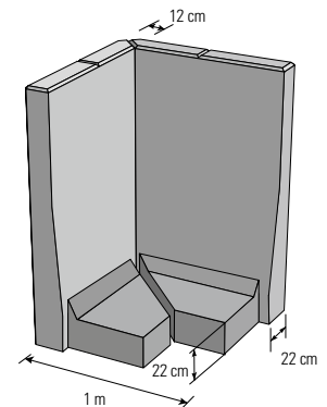
Mauerscheiben-Ecken Höhe 1,80 m–3,05 m
