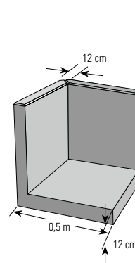
Mauerscheiben-Ecken Höhe 0,55 m–1,55 m
