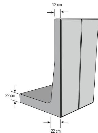
Mauerscheiben Höhe 1,80 m–3,05 m
