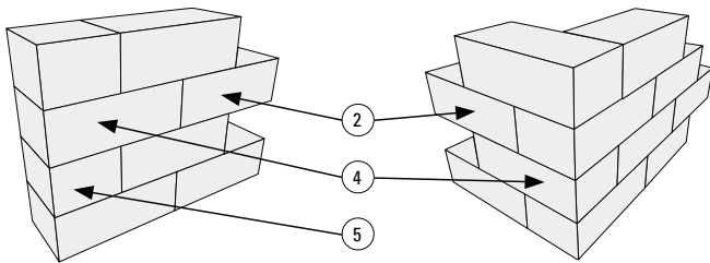
Aufbau der Vios-Mauer mit kleinformatischen Elementen (Halbversatz) Da alle Elemente auch auf der Oberseite feingestrahlt sind, werden diese auch als Abdecksteine verwendet.
