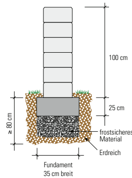
Freistehender Aufbau
