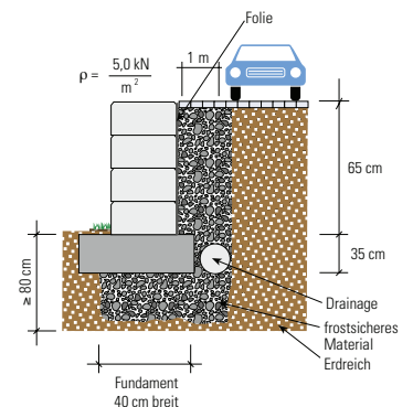
Senkrechter Aufbau, hinterfüllt, mit Verkehrslast
