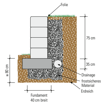
Senkrechter Aufbau, hinterfüllt, ohne Verkehrslast
