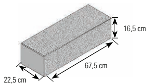
Typ 1: Grundelement groß Sichtflächen feingestrahlt, Köpfe un- bearbeitet, Oberseite feingestrahlt
