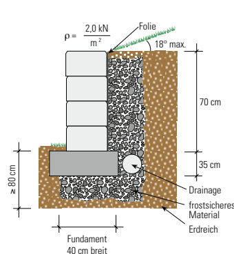
Senkrechter Aufbau, mit Böschung, hinterfüllt
