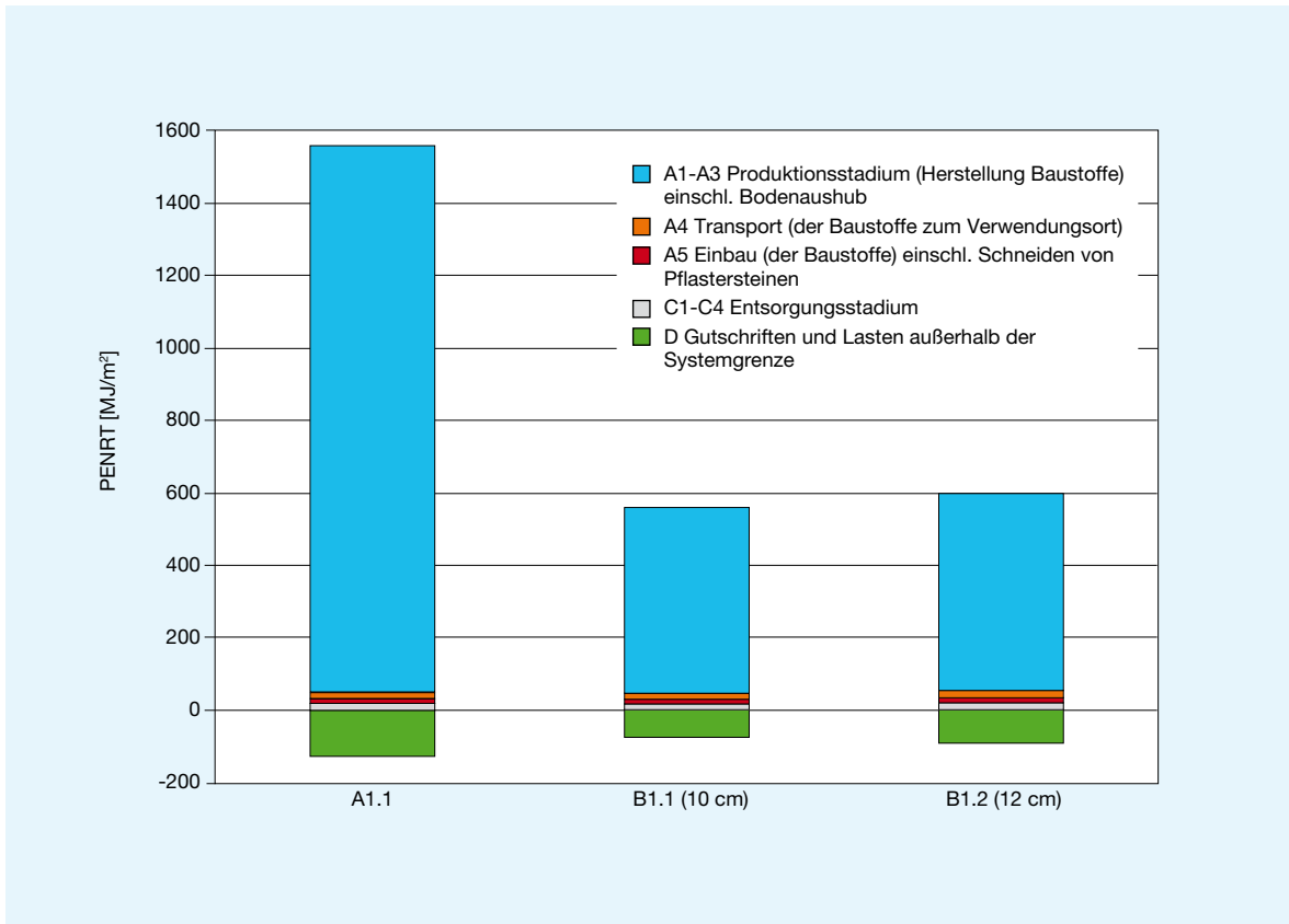
Abbildung 5-2: Ökobilanzergebnisse Beispiel 1, hier: nicht erneuerbarer Primärenergiebedarf PENRT in MJ/m²
