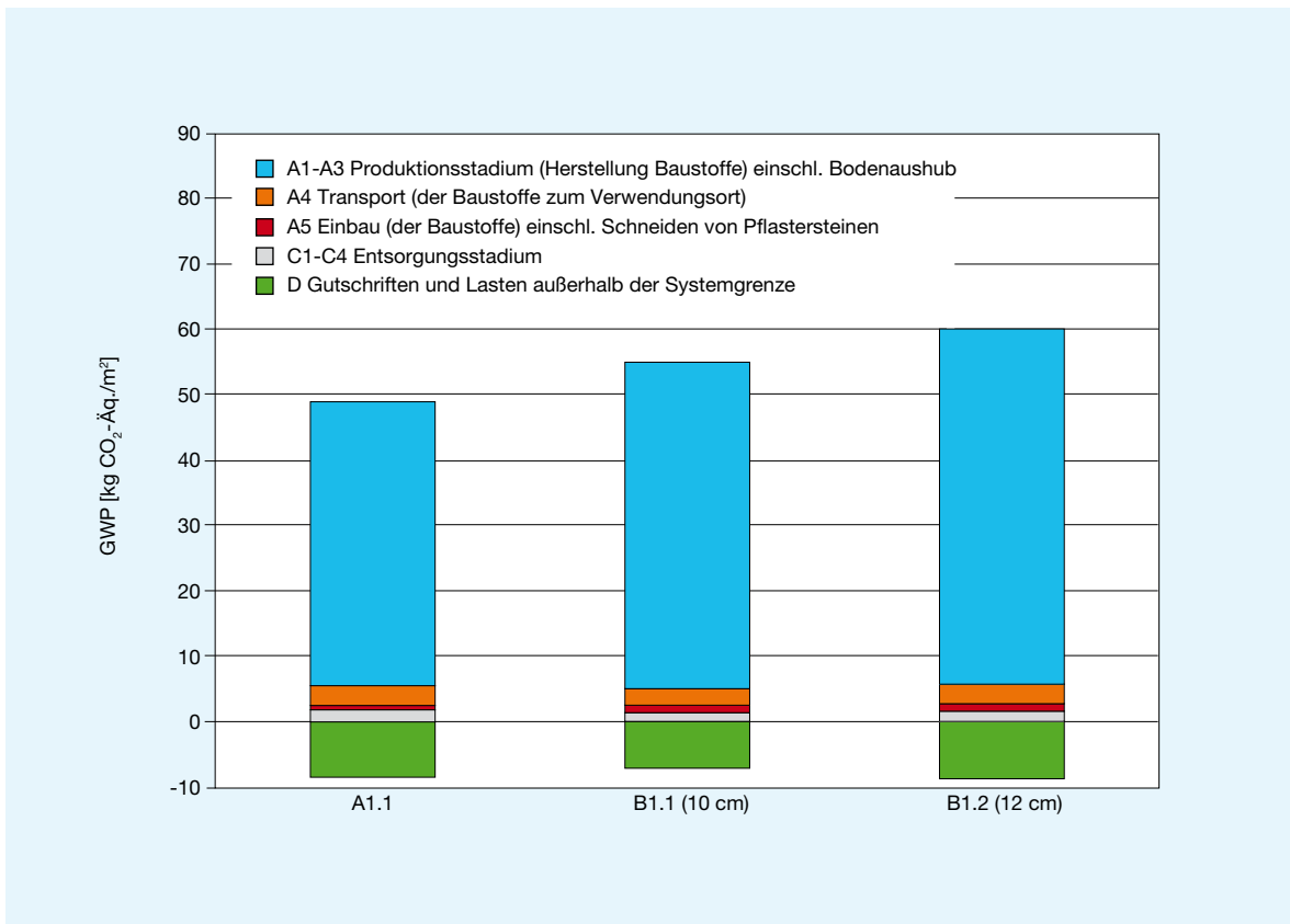
Abbildung 5-3: Ökobilanzergebnisse Beispiel 1, hier: Treibhauspotenzial GWP in kg CO₂-Äq./m²
