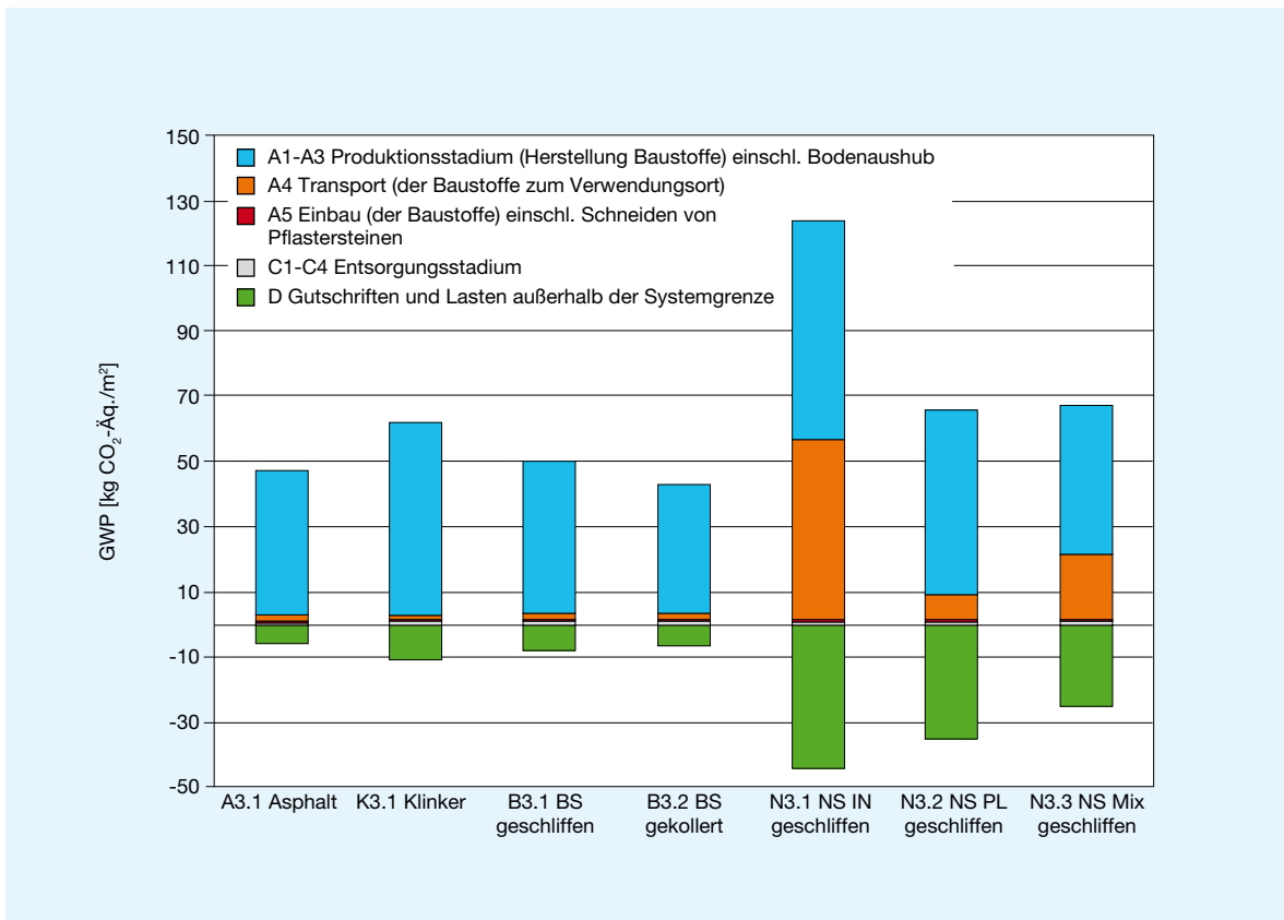
Abbildung 5-9: Ökobilanzergebnisse Beispiel 3, hier: Treibhauspotenzial GWP in kg CO₂-Äq./m²
