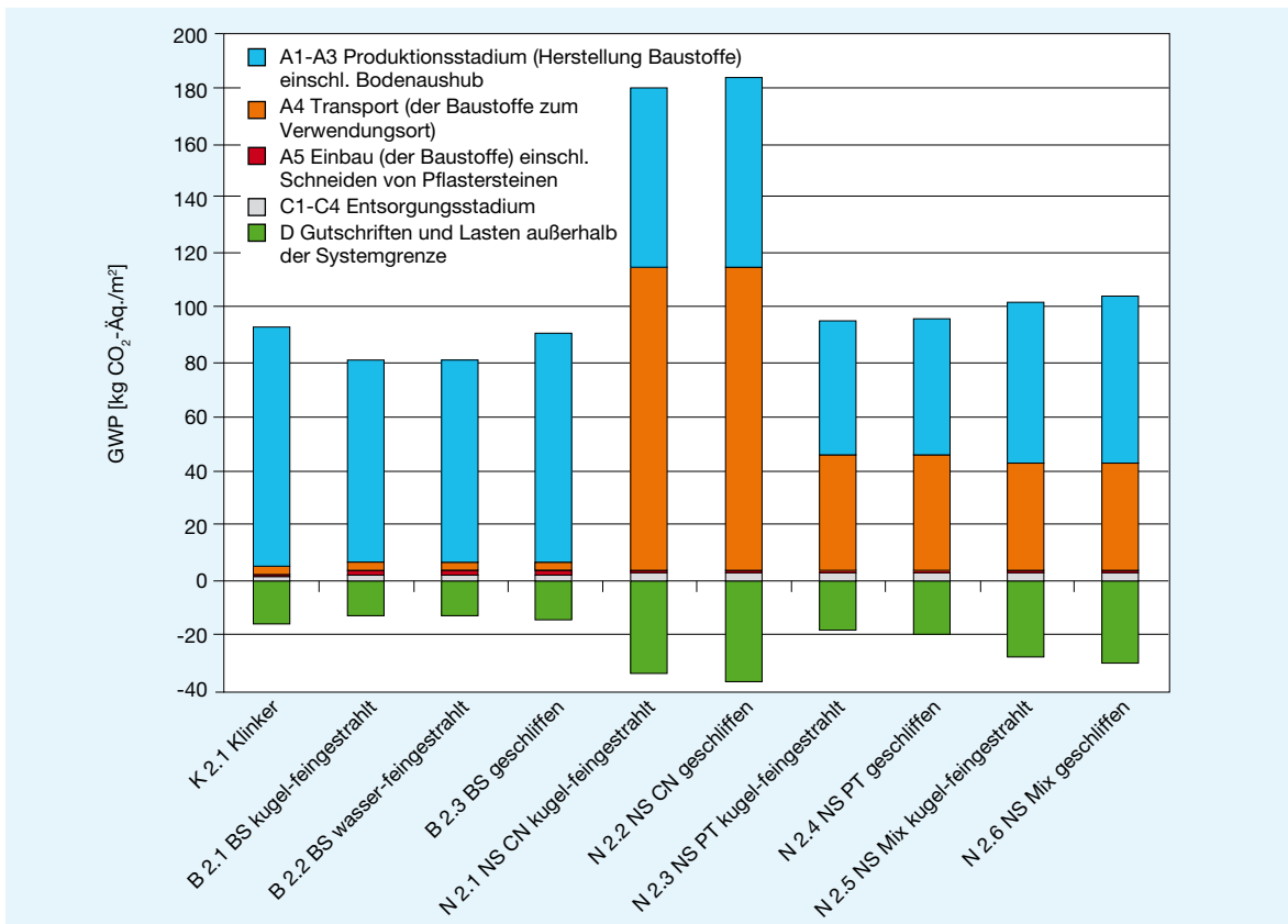
Abbildung 5-6: Ökobilanzergebnisse Beispiel 2, hier: Treibhauspotenzial GWP in kg CO 2 -Äq./m²
